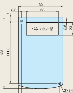
パネルカット寸法図 (矢視A)
