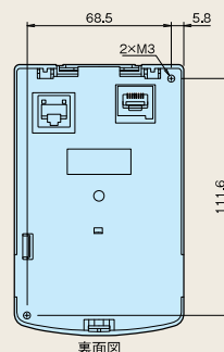
裏面図
