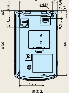
裏面図
