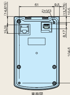
裏面図
